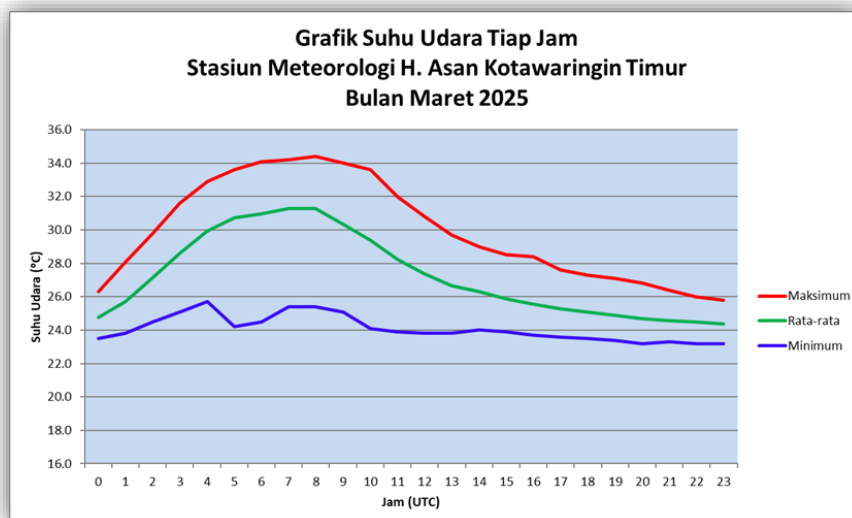
Gambar 1. Grafik Suhu Udara Tiap Jam Bulan Maret 2025
