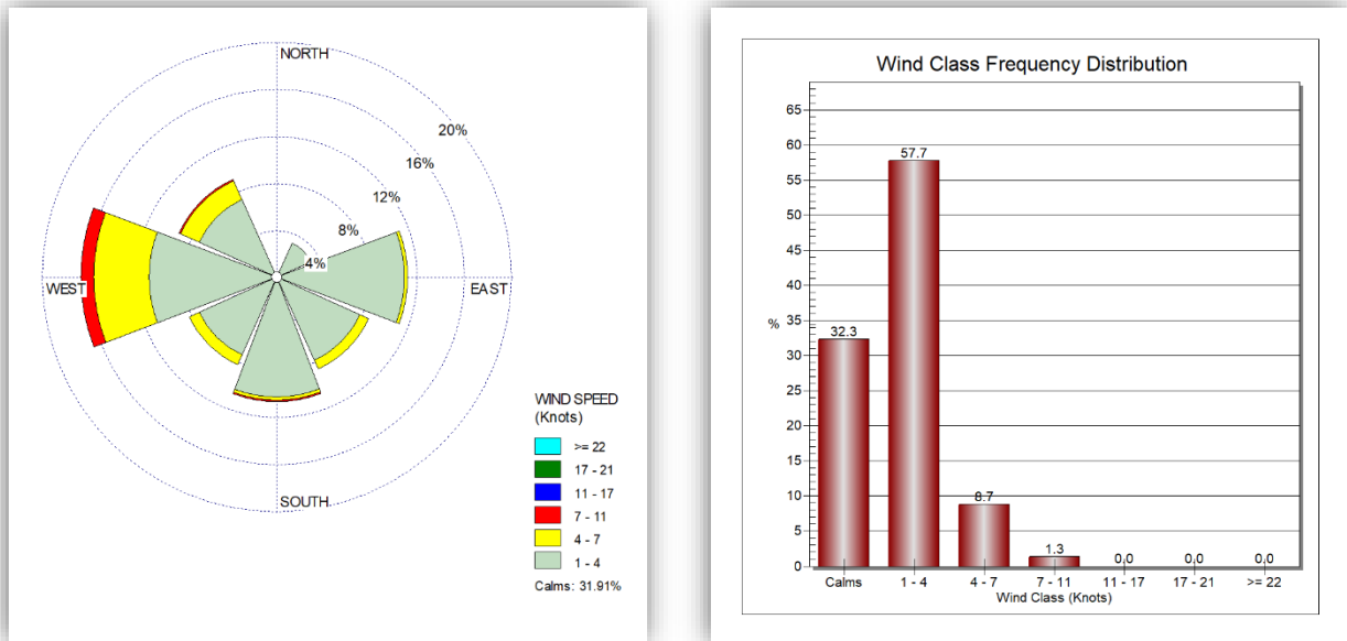
Gambar 8. Windrose dan Grafik Kecepatan Angin bulan Maret 2025
