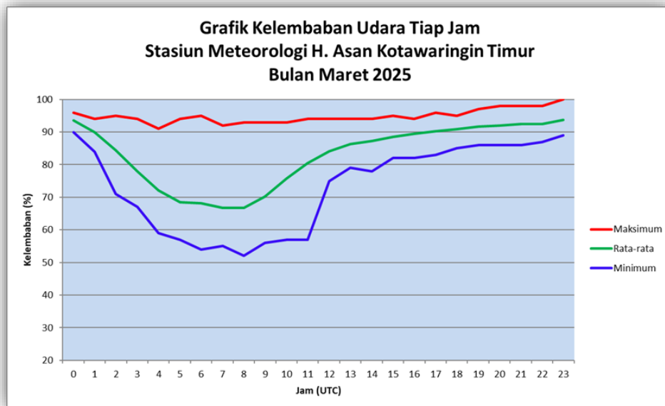
Gambar 3. Grafik Kelembaban Udara Tiap Jam Bulan Maret 2025
