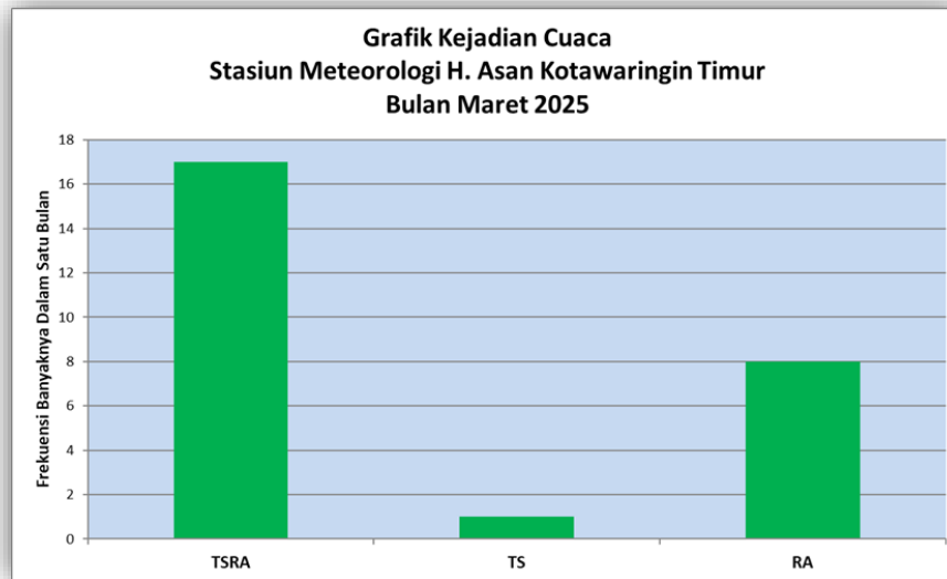
Gambar 9. Grafik Banyak Hari dan Kejadian Cuaca Khusus Bulan Maret 2025
