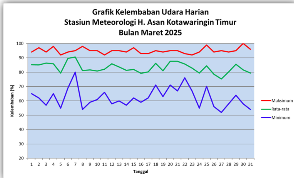
Gambar 4. Grafik Kelembaban Udara Harian Bulan Maret 2025
