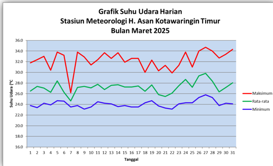
Gambar 2. Grafik Suhu Maksimum dan Suhu Minimum Harian Bulan Maret 2025
