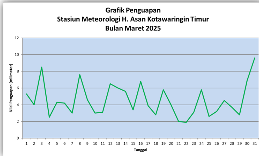
Gambar 5. Grafik Penguapan Harian Bulan Maret 2025
