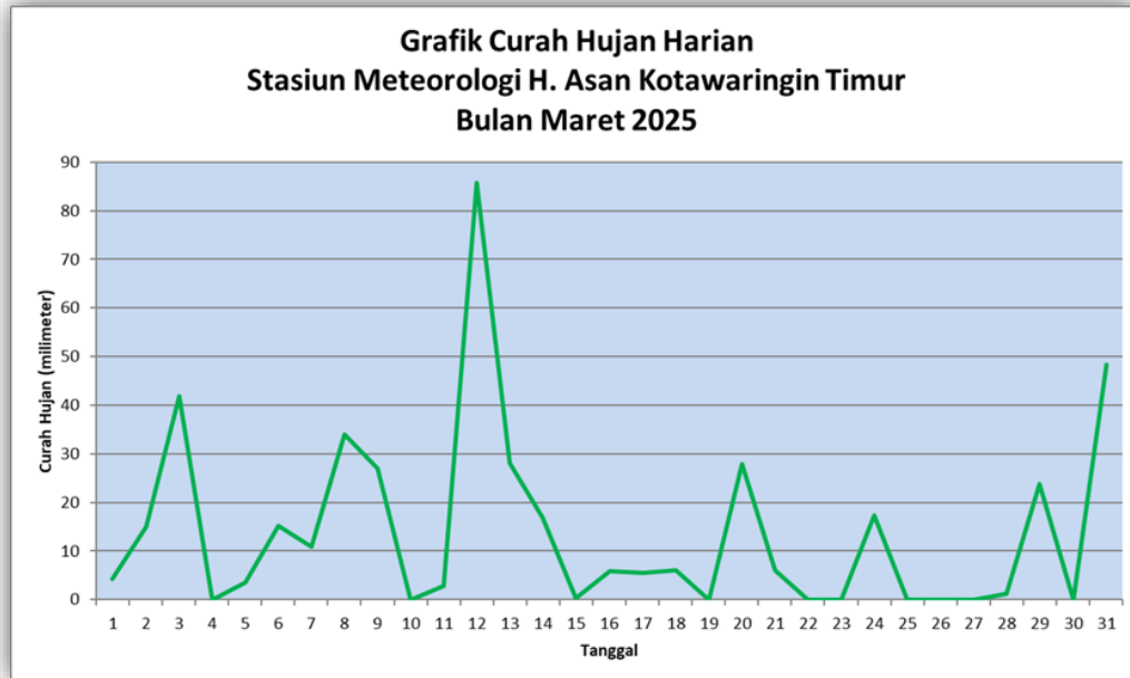
Gambar 6. Grafik Curah Hujan Harian Bulan Maret 2025
