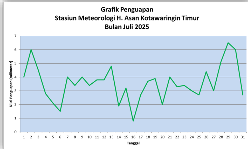
Gambar 5. Grafik Penguapan Harian Bulan Juli 2025
