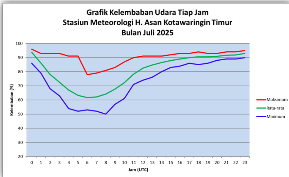
Gambar 3. Grafik Kelembaban Udara Tiap Jam Bulan Juli 2025
