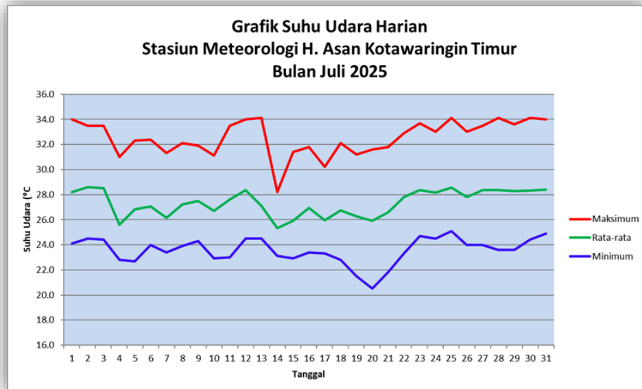
Gambar 2. Grafik Suhu Maksimum dan Suhu Minimum Harian Bulan Juli 2025
