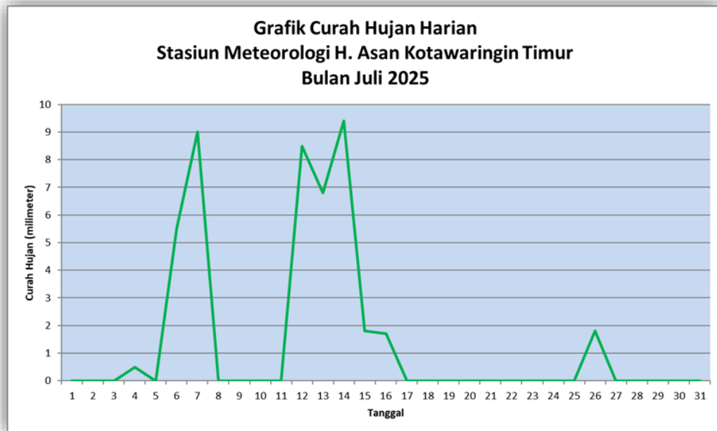
Gambar 6. Grafik Curah Hujan Harian Bulan Juli 2025
