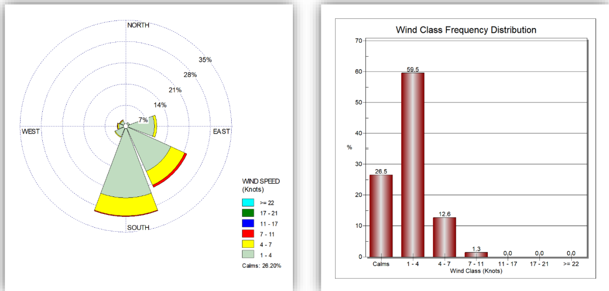
Gambar 8. Windrose dan Grafik Kecepatan Angin bulan Juli 2025
