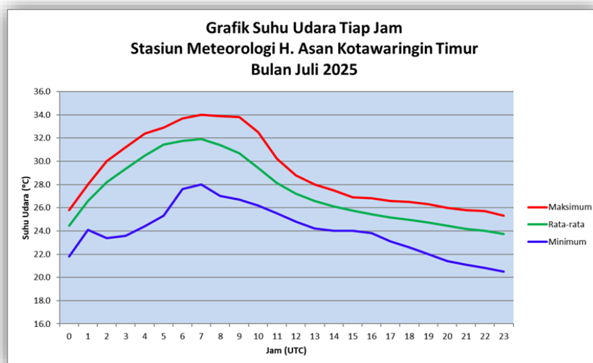
Gambar 1. Grafik Suhu Udara Tiap Jam Bulan Juli 2025
