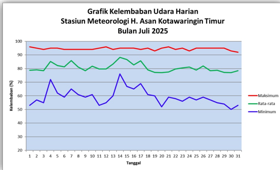
Gambar 4. Grafik Kelembaban Udara Harian Bulan Juli 2025
