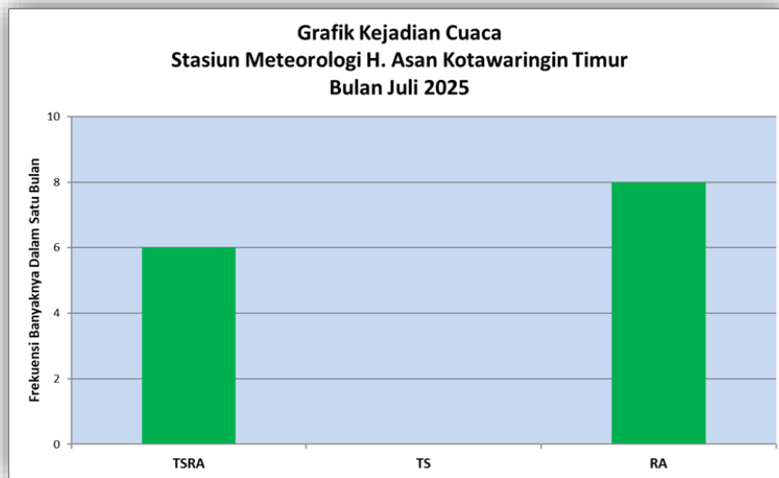
Gambar 9. Grafik Banyak Hari dan Kejadian Cuaca Khusus Bulan Juli 2025
