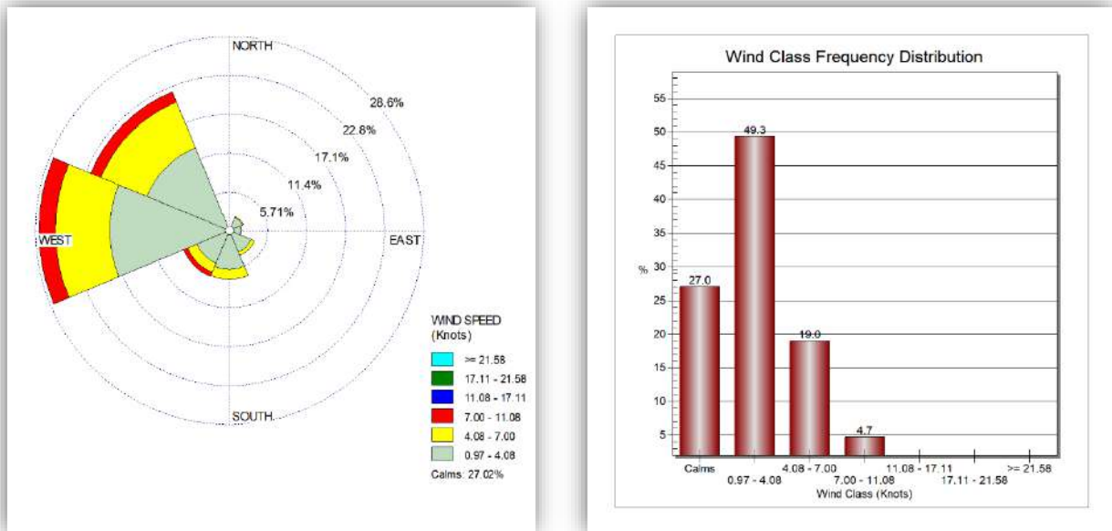
Gambar 8. Windrose dan Grafik Kecepatan Angin bulan Januari 2026
