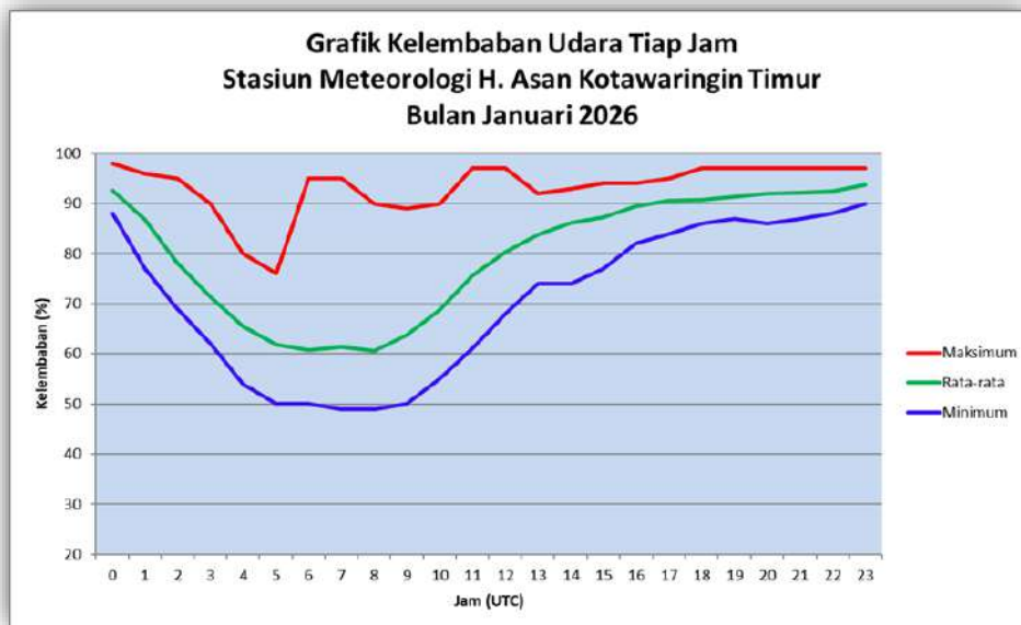
Gambar 3. Grafik Kelembaban Udara Tiap Jam Bulan Januari 2026
