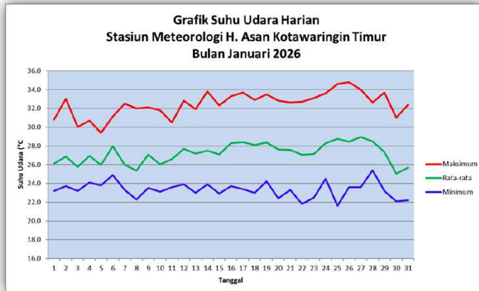
Gambar 2. Grafik Suhu Maksimum dan Suhu Minimum Harian Bulan Januari 2026
