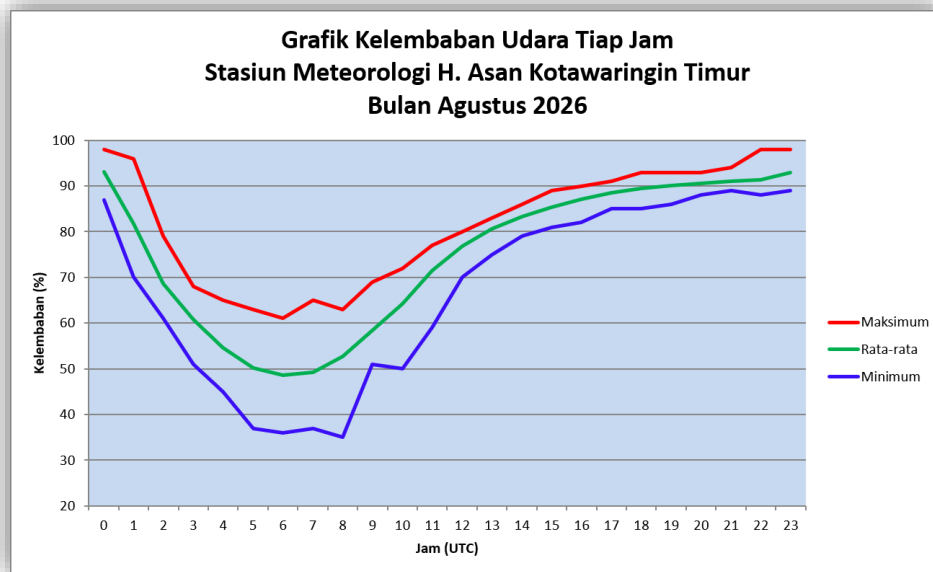
Gambar 3. Grafik Kelembaban Udara Tiap Jam Bulan Agustus 2026
