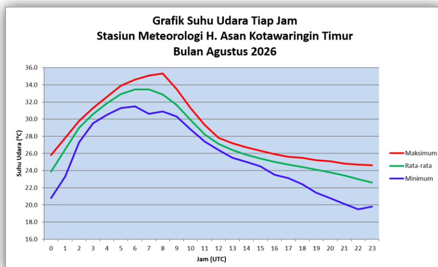
Gambar 1. Grafik Suhu Udara Tiap Jam Bulan Agustus 2026
