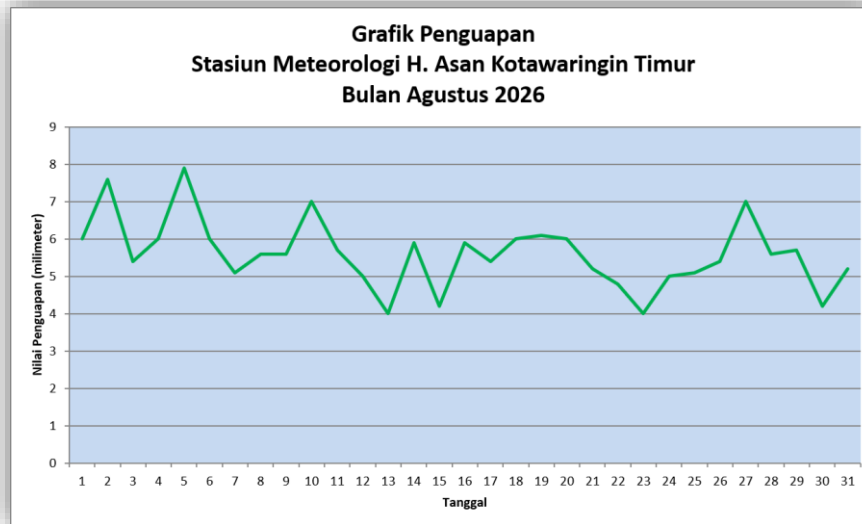
Gambar 5. Grafik Penguapan Harian Bulan Agustus 2026
