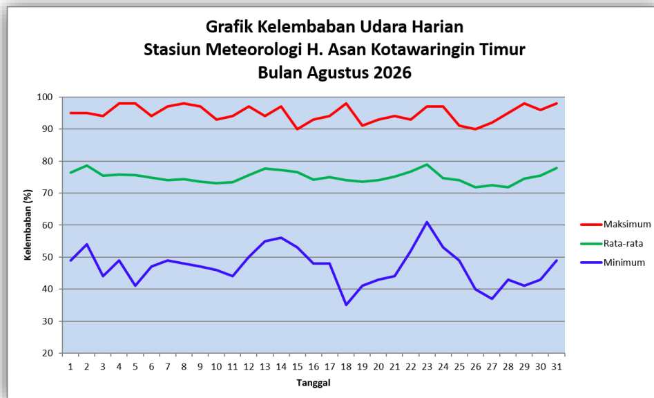
Gambar 4. Grafik Kelembaban Udara Harian Bulan Agustus 2026
