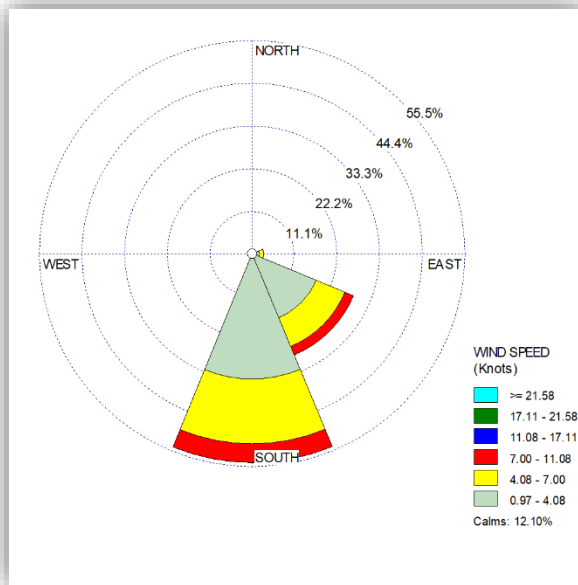
Gambar 8. Windrose dan Grafik Kecepatan Angin bulan Agustus 2026
