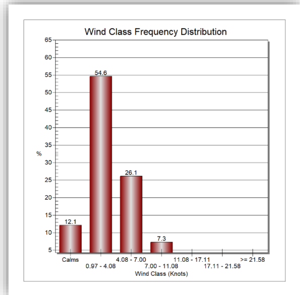
Gambar 8. Windrose dan Grafik Kecepatan Angin bulan Agustus 2026
