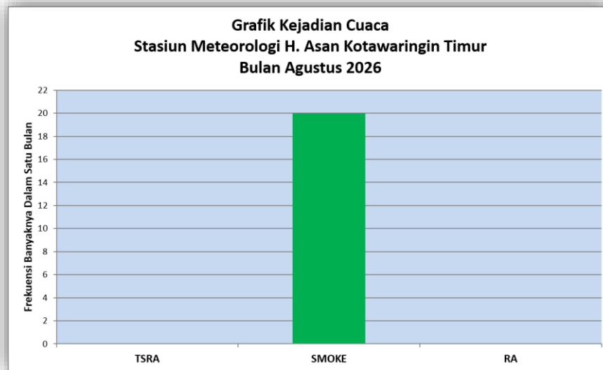
Gambar 9. Grafik Banyak Hari dan Kejadian Cuaca Khusus Bulan Agustus 2026
