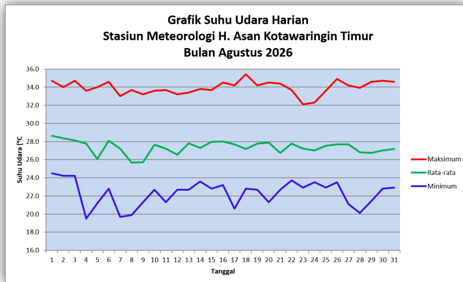
Gambar 2. Grafik Suhu Maksimum dan Suhu Minimum Harian Bulan Agustus 2026
